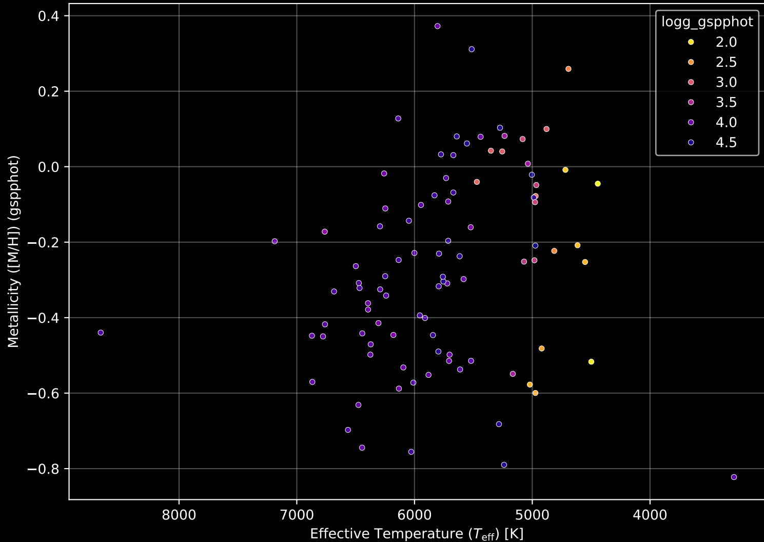
GALAH DR4 Field: [7181] Stellar Population Parameters (n= 95)
