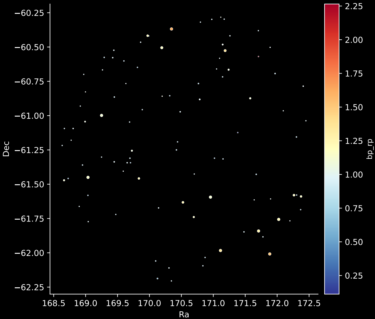
GALAH DR4 Field: [7181] Stars: 95
